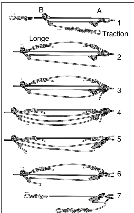
Fig 49 – Inversion montée descente
