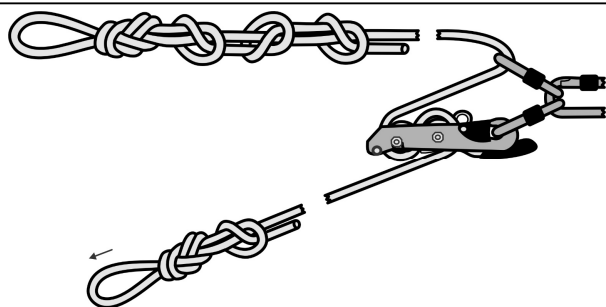
Fig. 44 – Frein de charge
